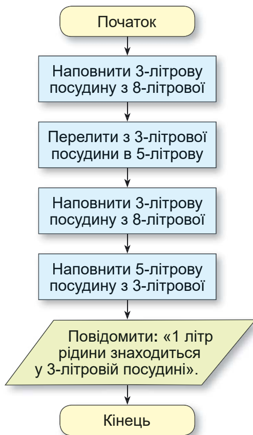
Мал. 5.14. Блок-схема алгоритму отримання 1 л рідини
