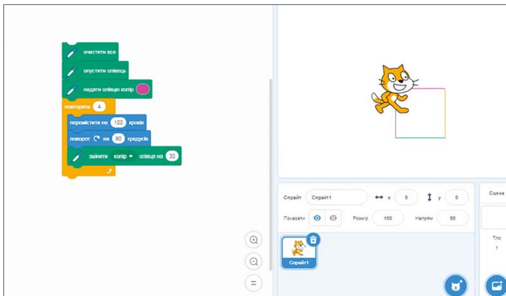
Мал. 5.44. Проект малювання різнокольорового квадрата зі змінням кольорів малювання в циклі
