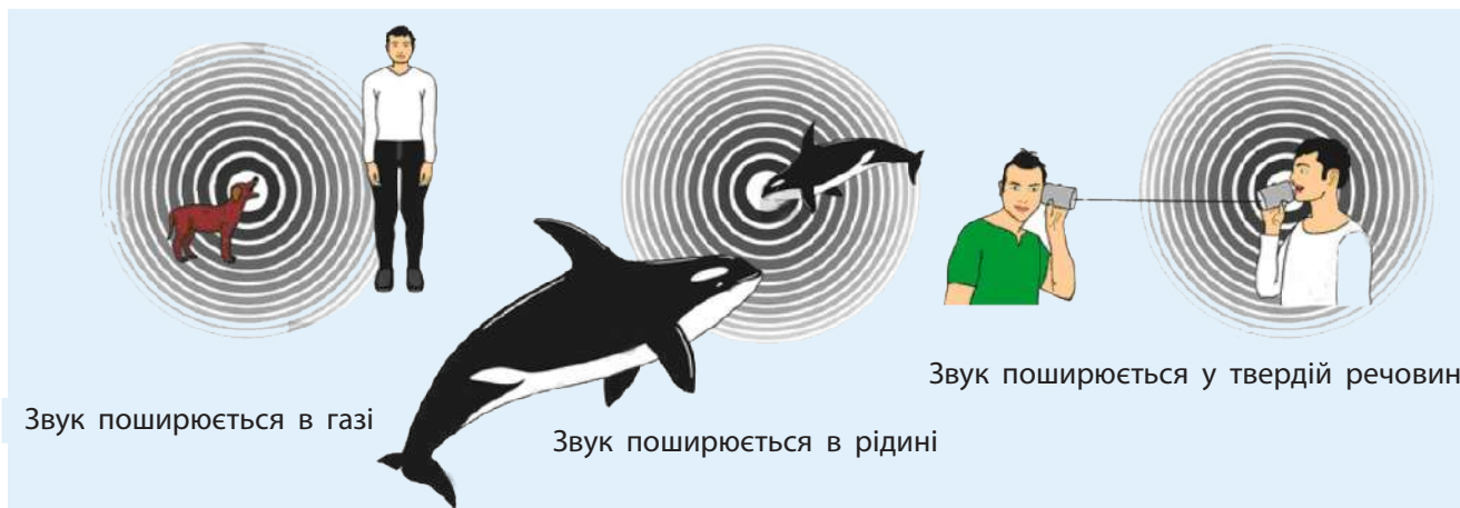
Мал. 42.2. Поширення звуку в різних середовищах
