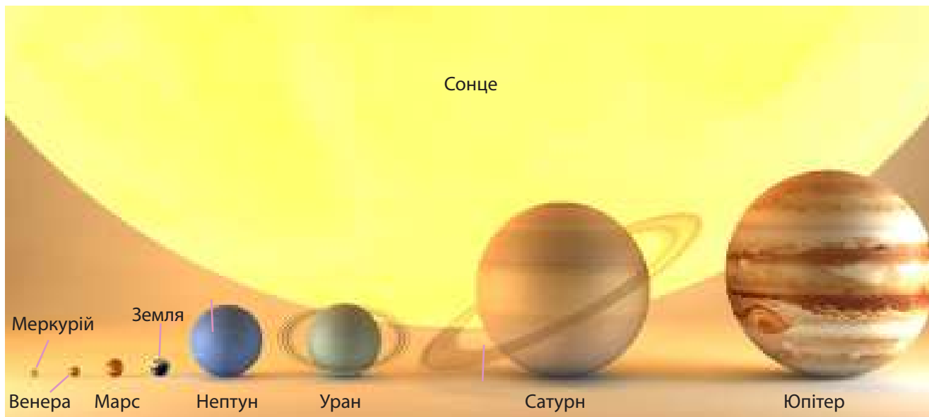
Мал. 15.2. Порівняння розмірів планет і Сонця
