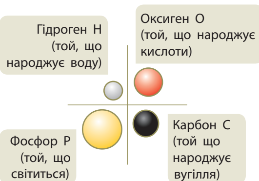
Мал. 2.2. Атоми та хімічні елементи
